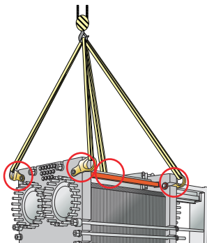
Joonis 7: Tõsteseade T50 jaoks. Kindlustusseadmeid on vaja.
