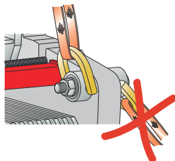
Joonis 8: Tõsteseade TS50 jaoks. Kasutage plaatsoojusvaheti tõstmisel nelja sisemist silmust. ÄRGE kasutage transportimiseks mõeldud kindlustuspunkte! Kindlustusseadmeid on vaja.
